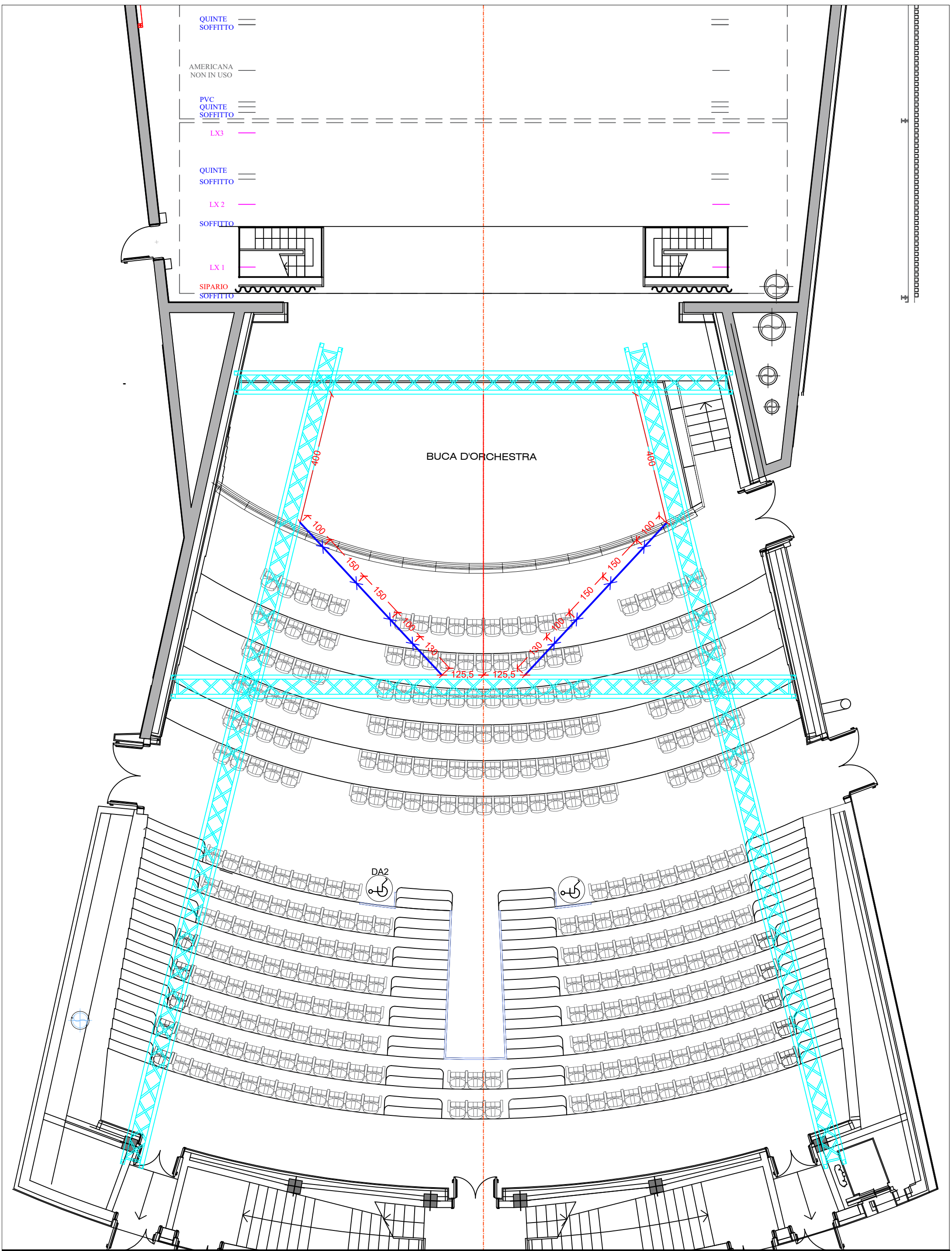
TEATRO LIRICO DI CAGLIARI PIANTA PLATEA TEATRO CARMEN MELIS SCALA 1:100
